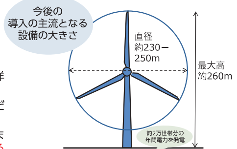
洋上風力発電（15MW級）
