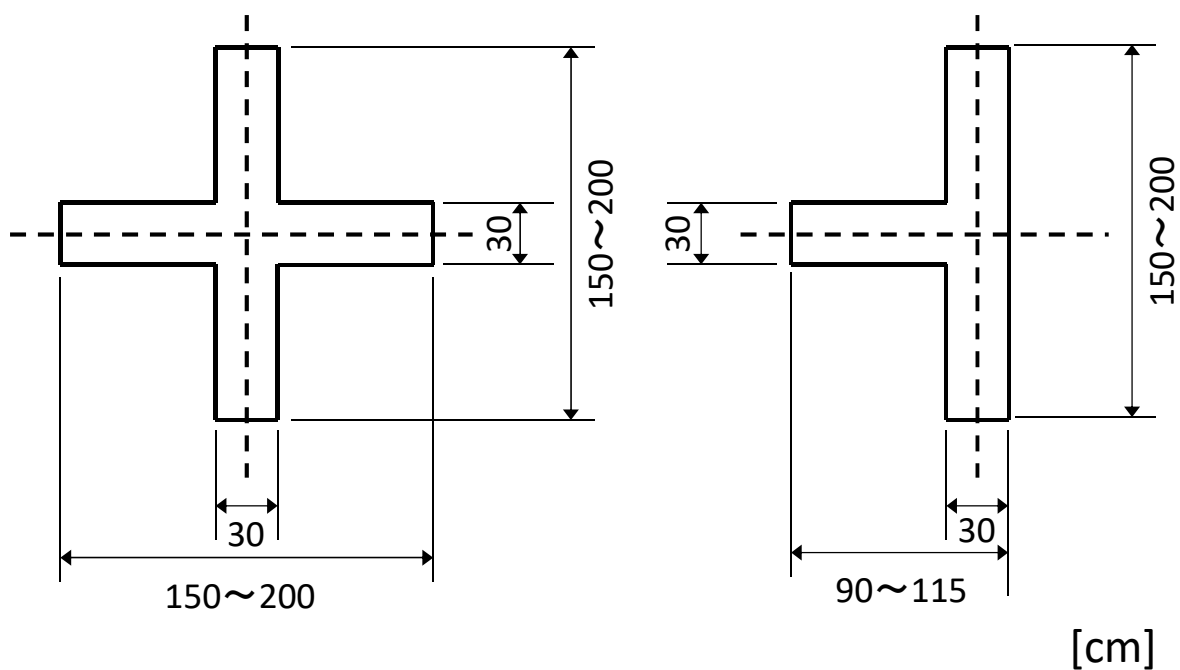
寸法図
