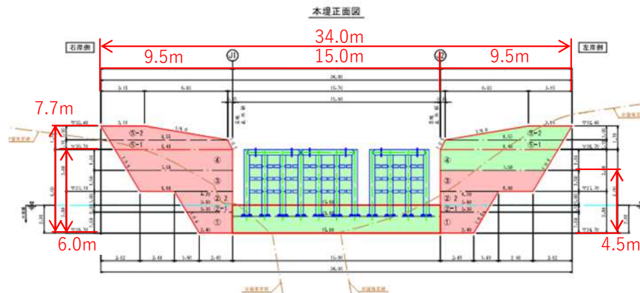
砂防えん堤(ダム) 正面図
