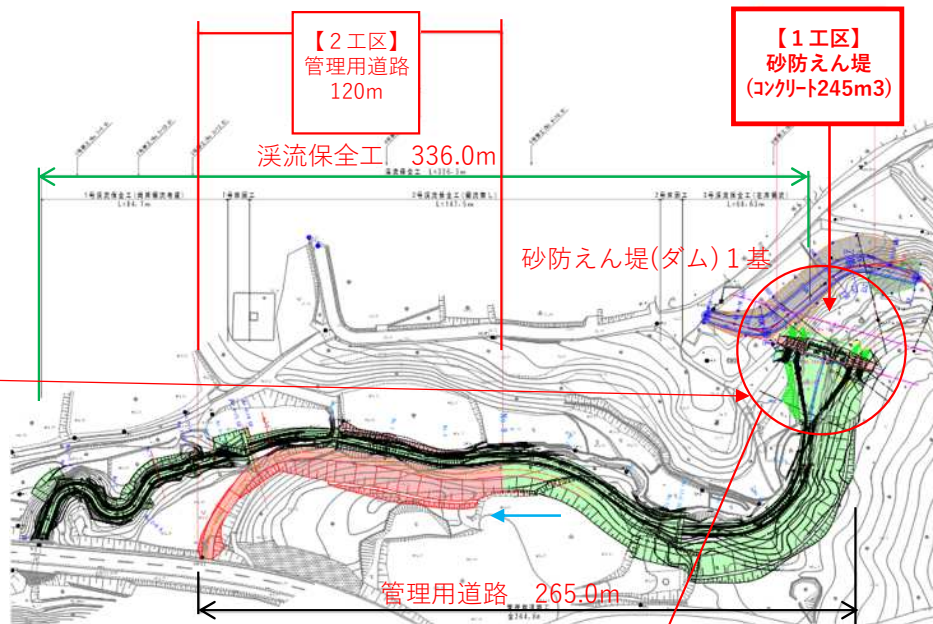
全体平面図
