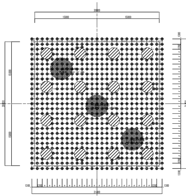
平面図（底版補修用吊足場） S=1:200
