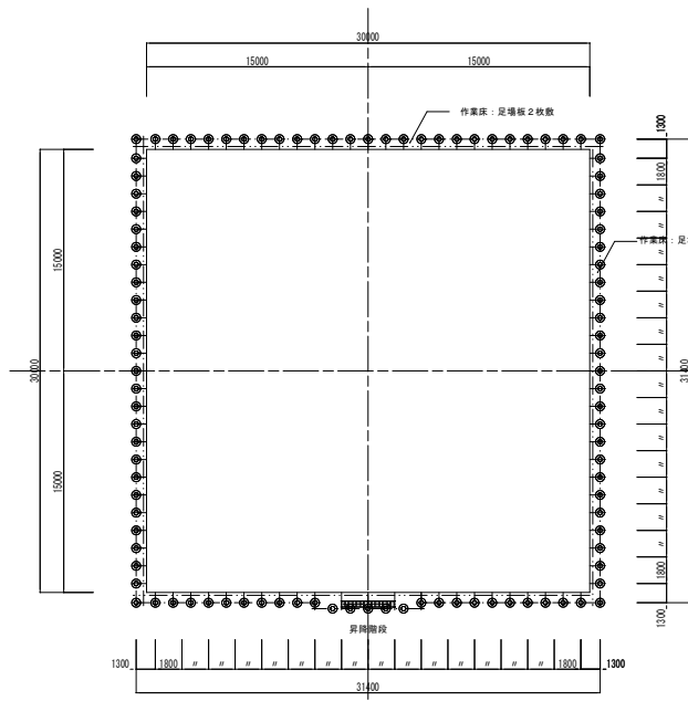
平面図（側面補修用吊足場） S=1:200
