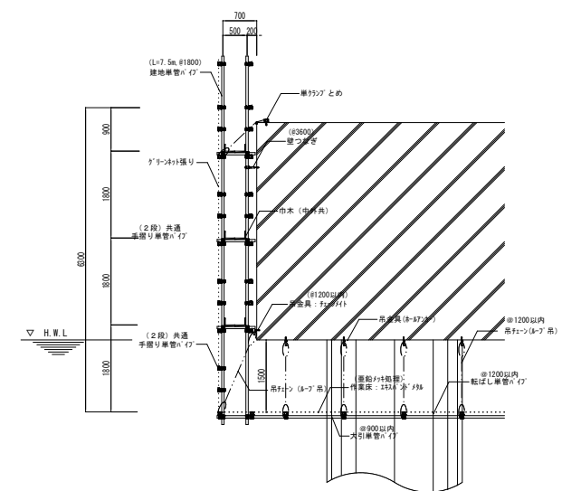
断面詳細図 S=1:50
