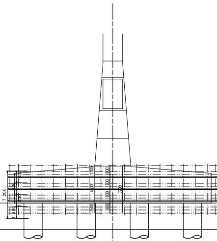
側面図 (P3側) S=1 : 200
