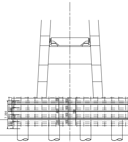
背面図（伊唐島側） S=1 : 200
