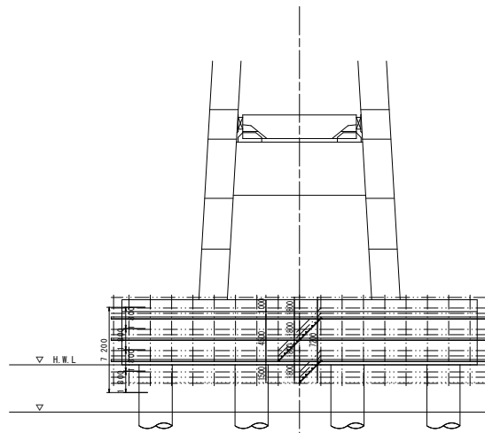
正面図（長島側） S=1 : 200
