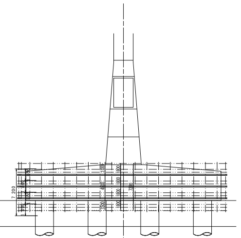
側面図 (P5側) S=1 : 200
