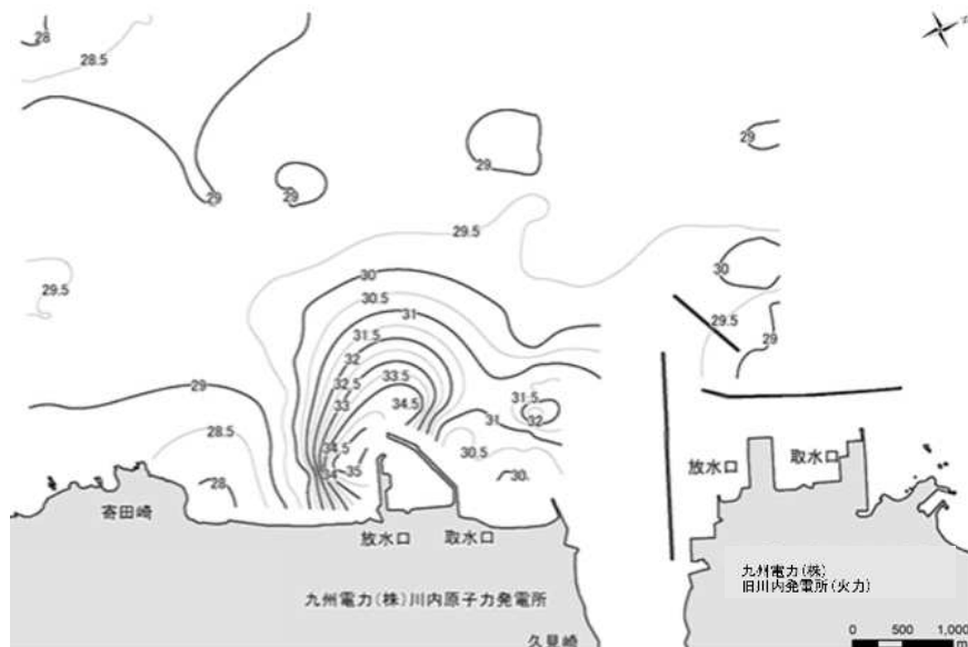
図10-1 表層(0.3m深)水温水平分布（上げ潮時） 単位：℃
