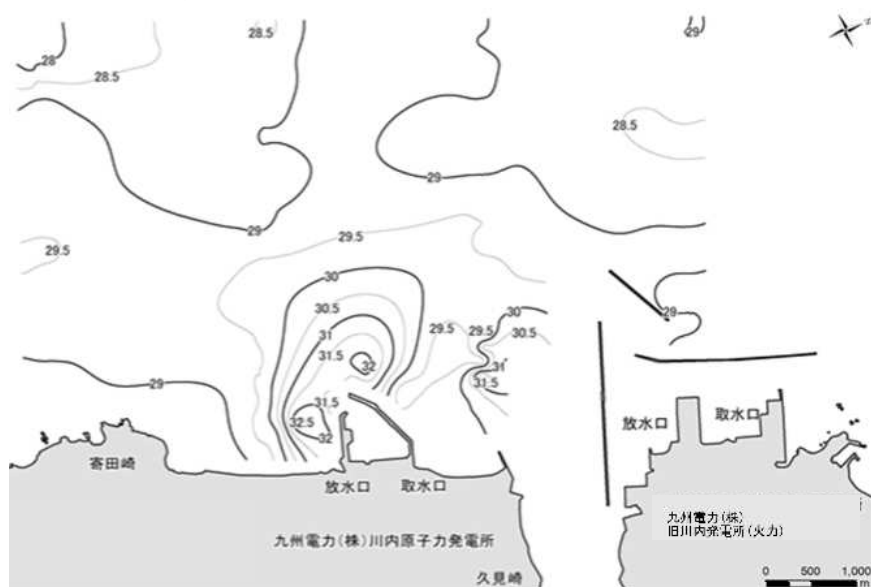
図10-2 1m層水温水平分布（上げ潮時） 単位：℃
