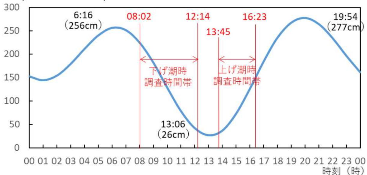
図7 水温・塩分水平分布調査日（令和6年7月20日）の潮汐（阿久根験潮場）と調査時間
