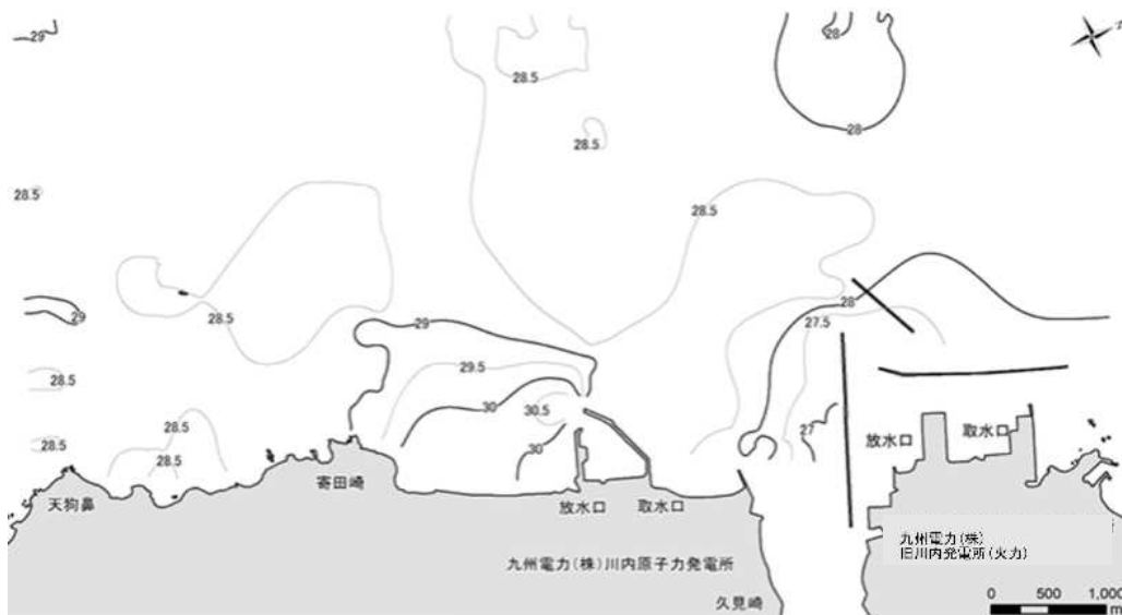
図9-2 1m層水温水平分布（下げ潮時） 単位：℃
