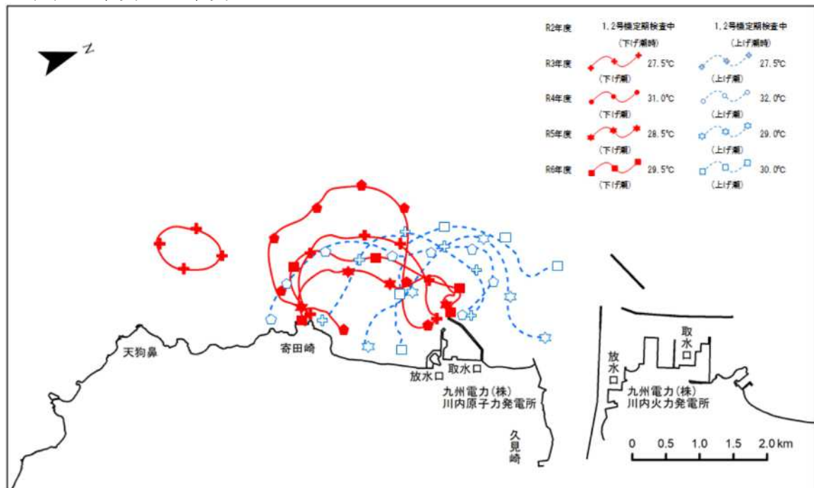
図12-10 令和2～6年度夏季表層(0.3m深)温排水拡散範囲
