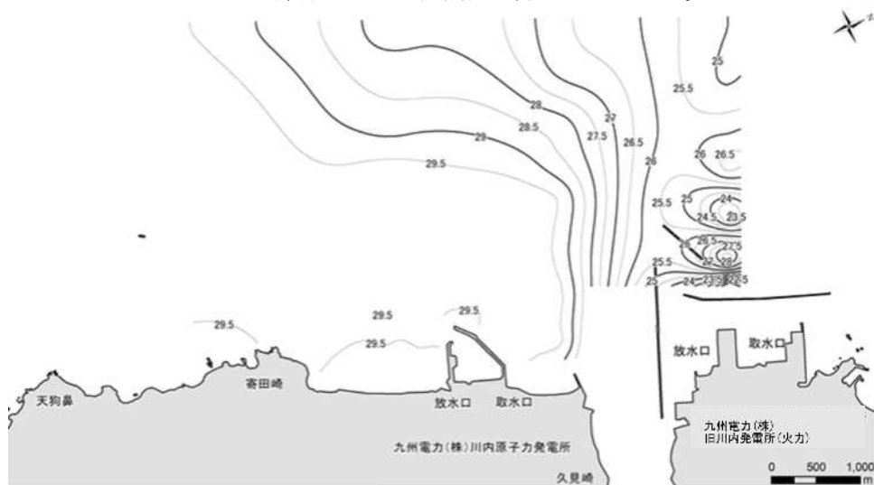
図11-2 表層(0.3m深)塩分水平分布(上げ潮時)
