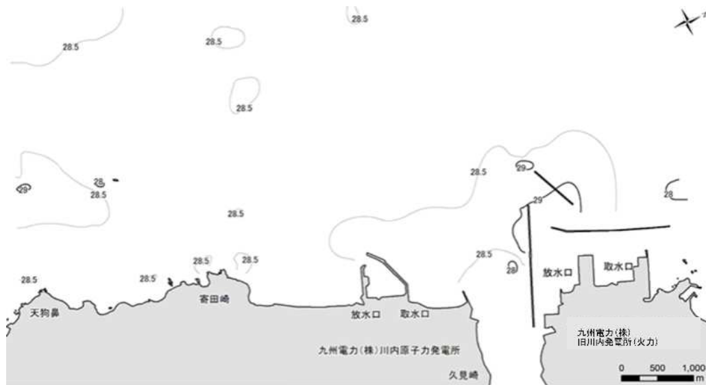
図 9-3 2m層水温水平分布（下げ潮時）
