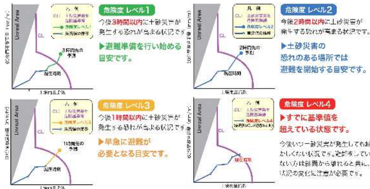
付図1 レベル土砂災害危険情報の発表及び解除基準
