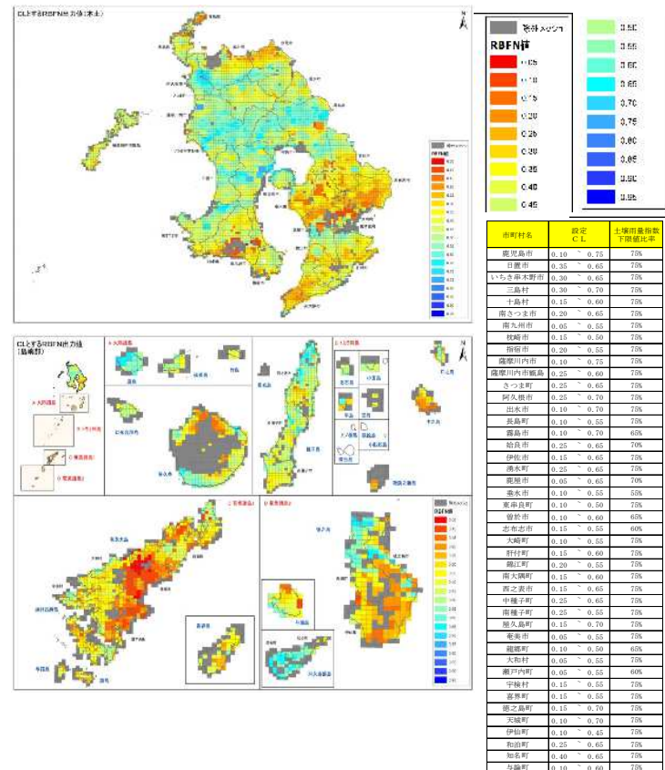
付図3 レベル4土砂災害危険情報の監視基準
