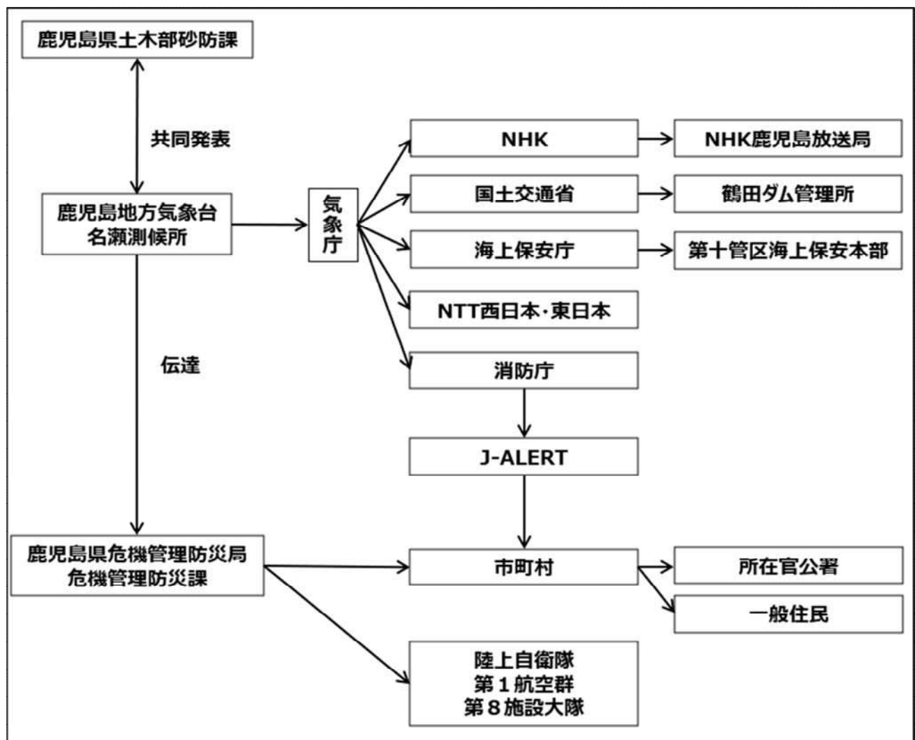
図3. 2. 1. 8 レベル4土砂災害危険警報の伝達系統図
