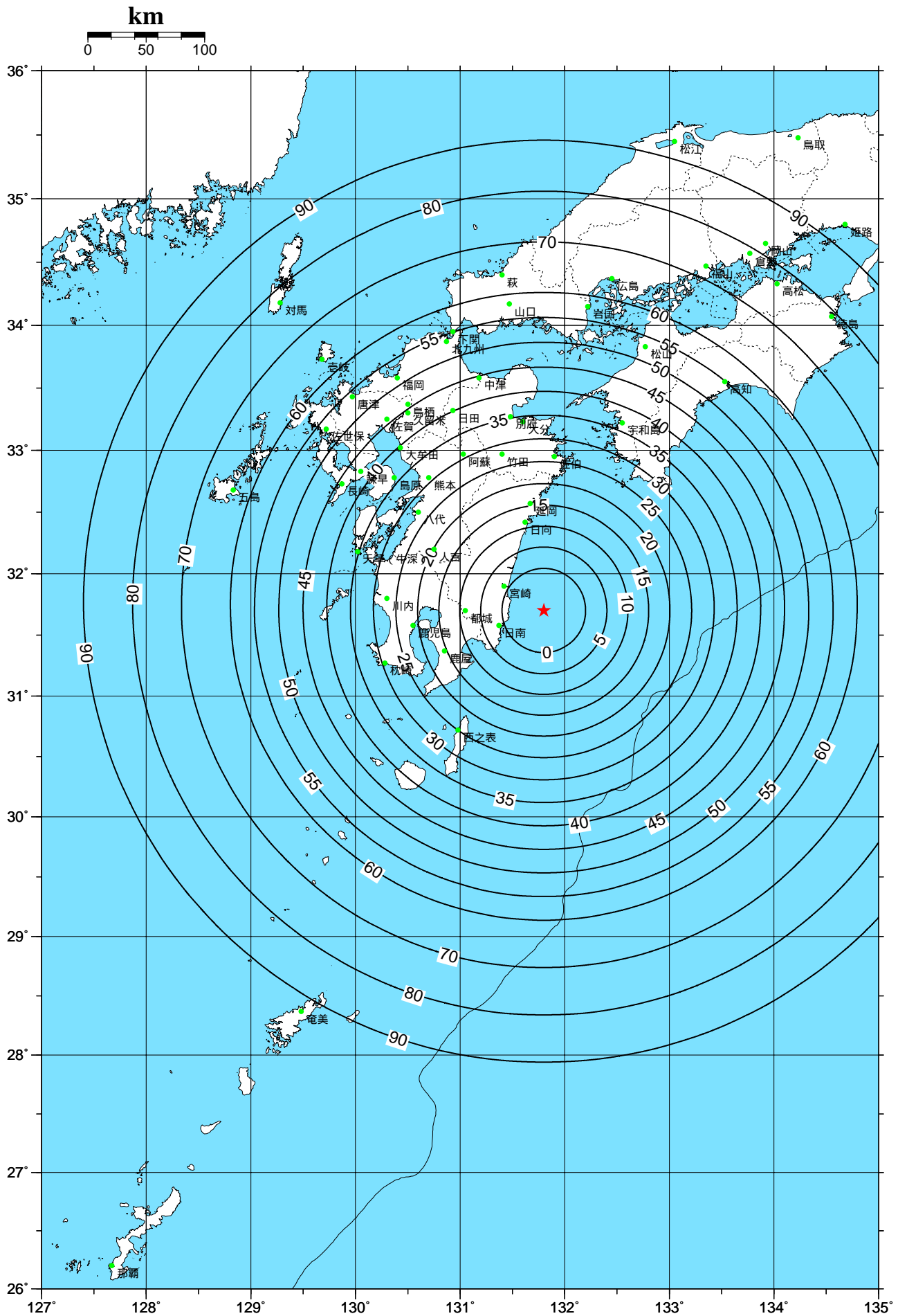
本図は、想定震源の座標（緯度・経度・深さ）を与え、最寄の観測点で地震波を検知した後、5秒後に緊急地震速報を発信したと仮定して、主要動到達までの猶予時間を描画したものである。なお、本図は理論計算値に基づくものであるため、実際の地震の場合はこれと異なることに留意が必要である。
