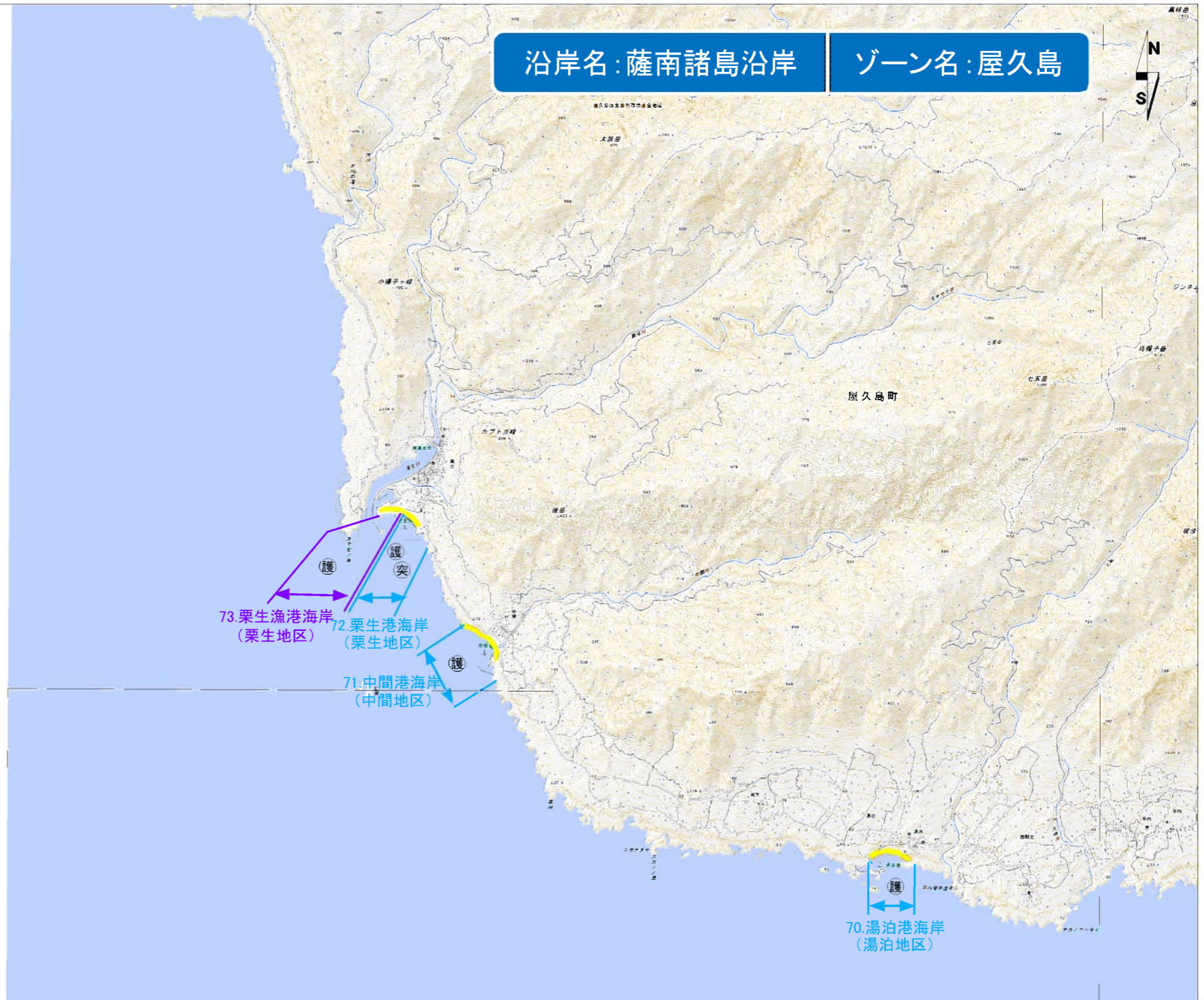
図 海岸保全施設の整備区域、種類、規模及び配置 29/56
