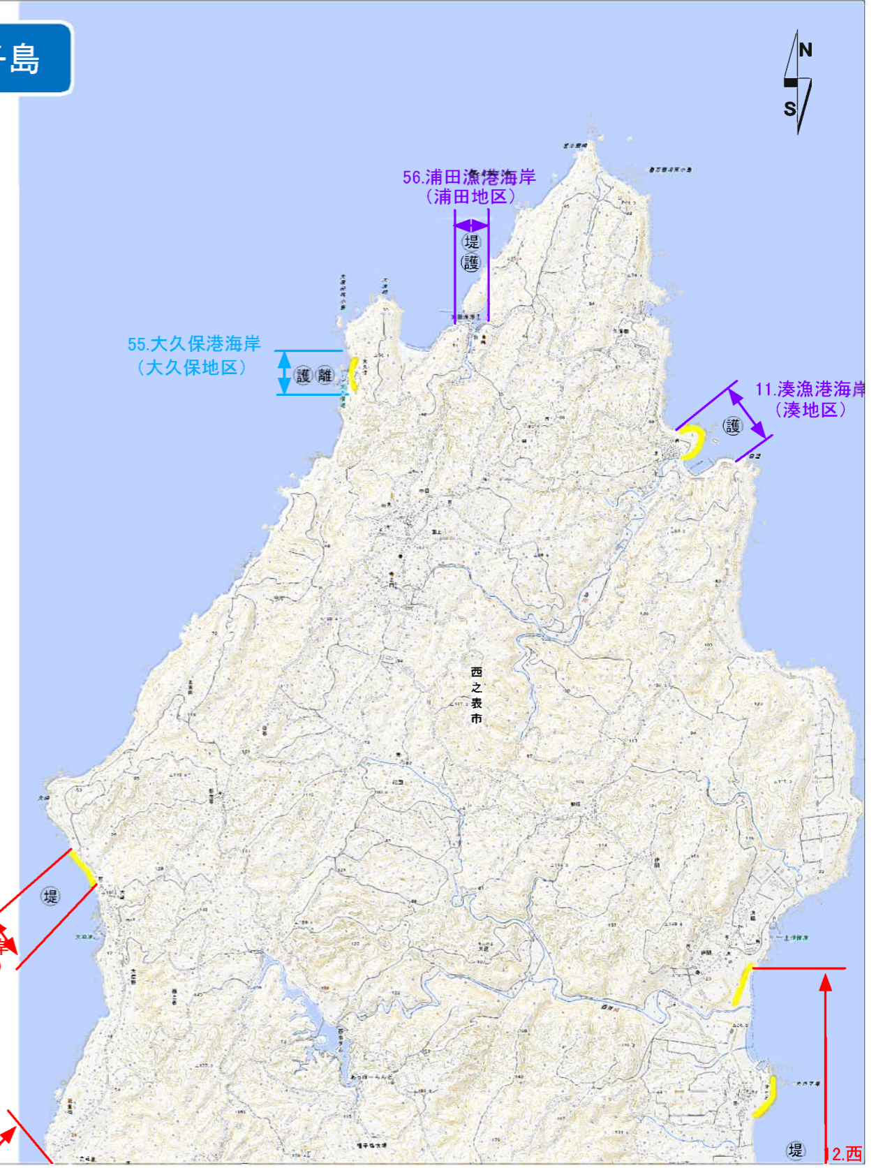
図 海岸保全施設の整備区域、種類、規模及び配置 24/56
