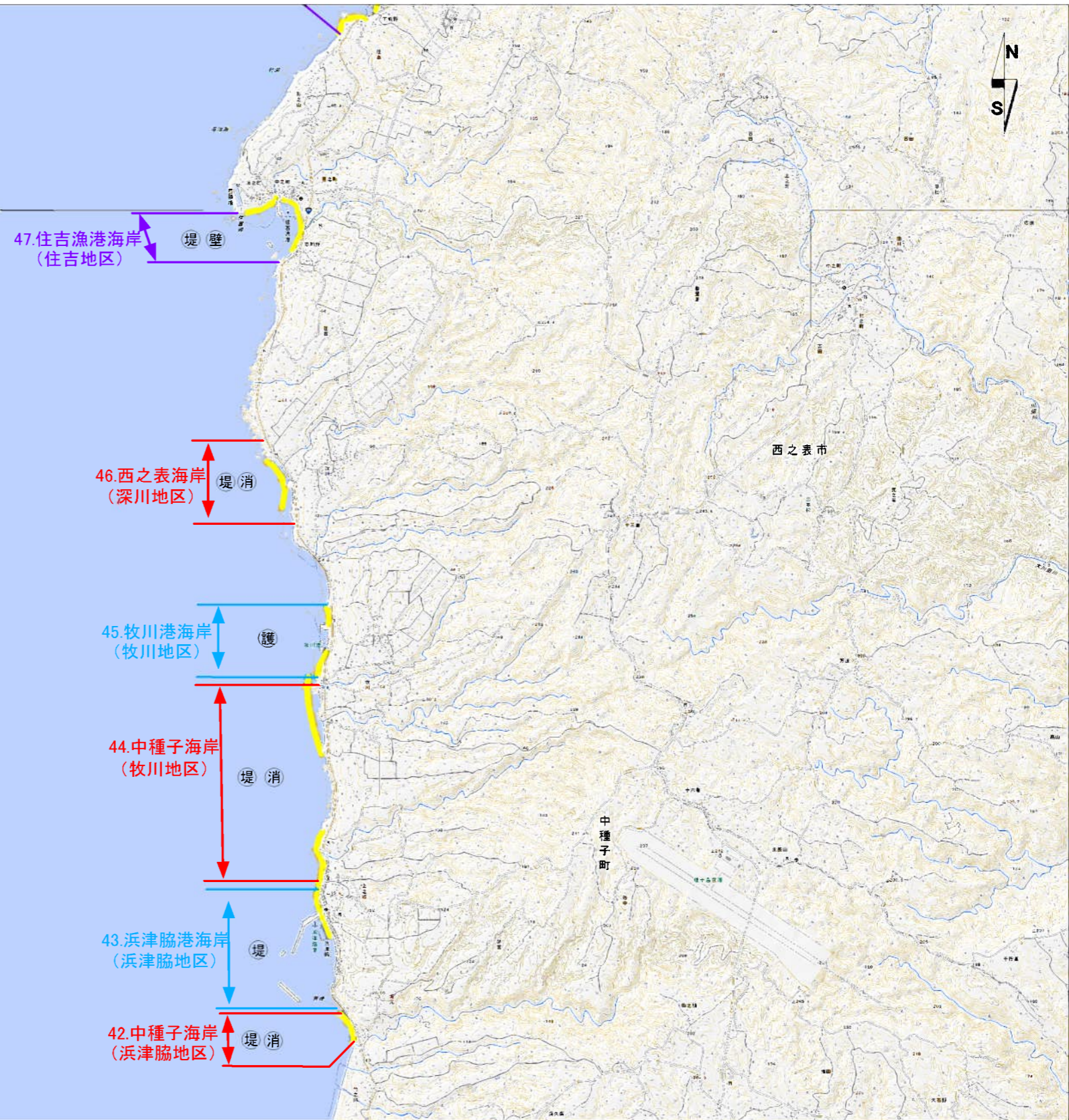
図 海岸保全施設の整備区域、種類、規模及び配置 22/56
