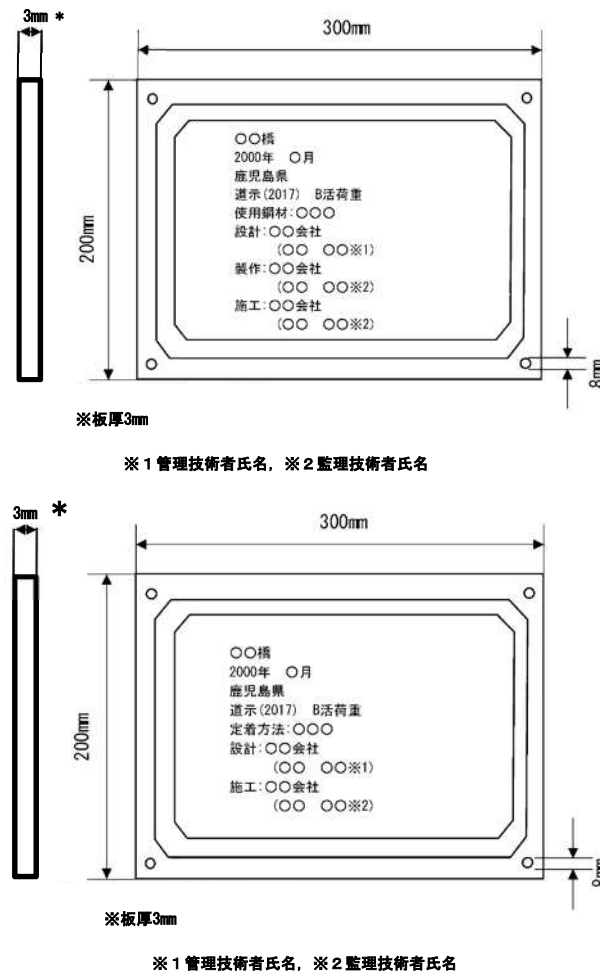
図3-2-2 銘板の寸法及び記載事項
