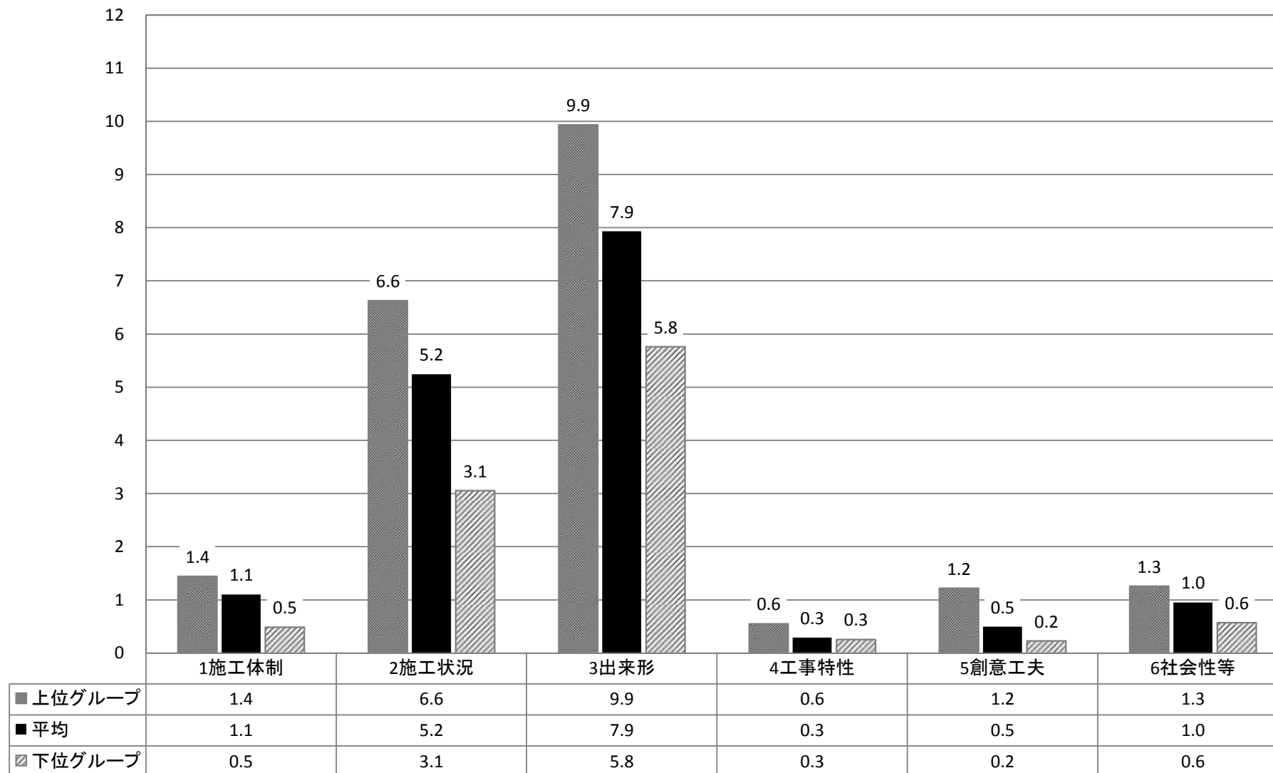
図2-3 考査項目1～6の平均値と上下グループ間の差（H28年度完成 土木部発注の土木一式工事）
