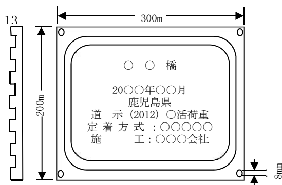
板厚 8mm，字厚 5mm，計 13mm
