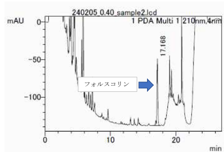
図3 標準溶液のクロマトグラム (抜粋)
