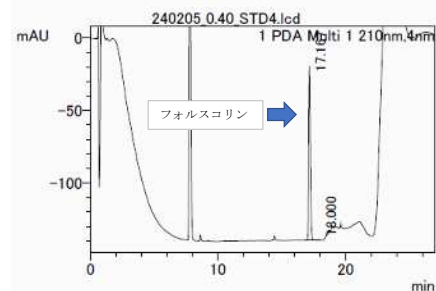
図2 試料溶液のクロマトグラム (抜粋)
