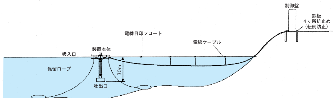
図1-22 池田湖水質改善実験
