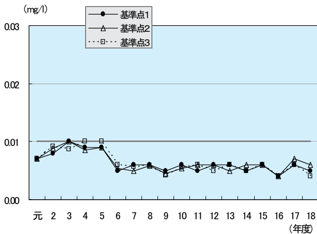
図 1-18 全りん (T-P)
