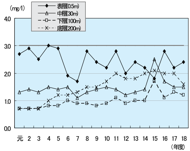
図 1-16 COD
