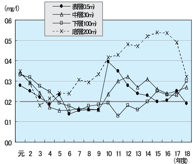
図 1-17 全窒素 (T-N)
