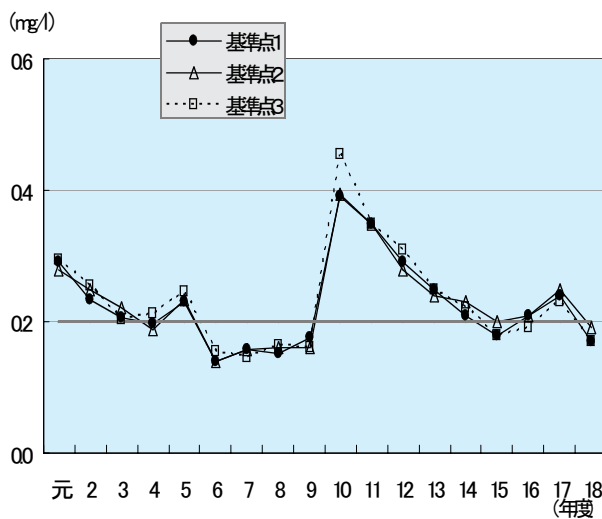
図 1-17 全窒素 (T-N)
