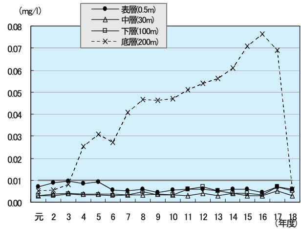
図 1-18 全りん (T-P)
