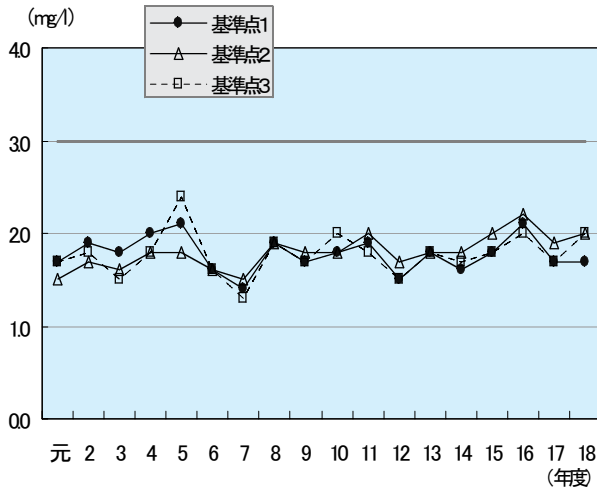
図 1-16 COD
