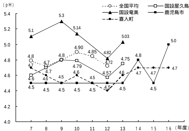
図1-7 年平均値（pH）の推移
