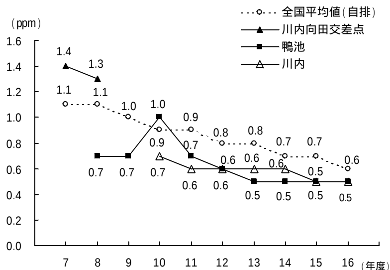
図 1 - 6 一酸化炭素の年平均値の推移
